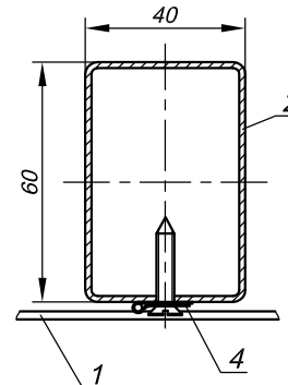
Крепление - зажим/саморез
